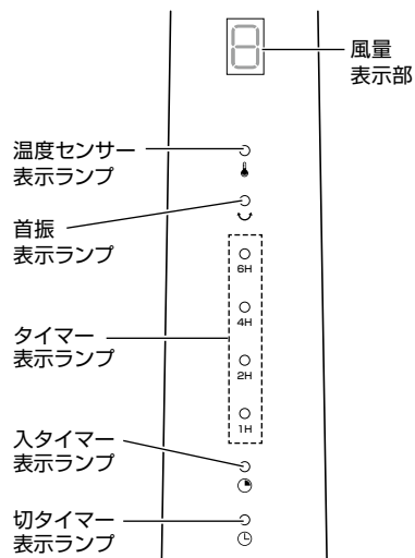
本体：表示部拡大図
