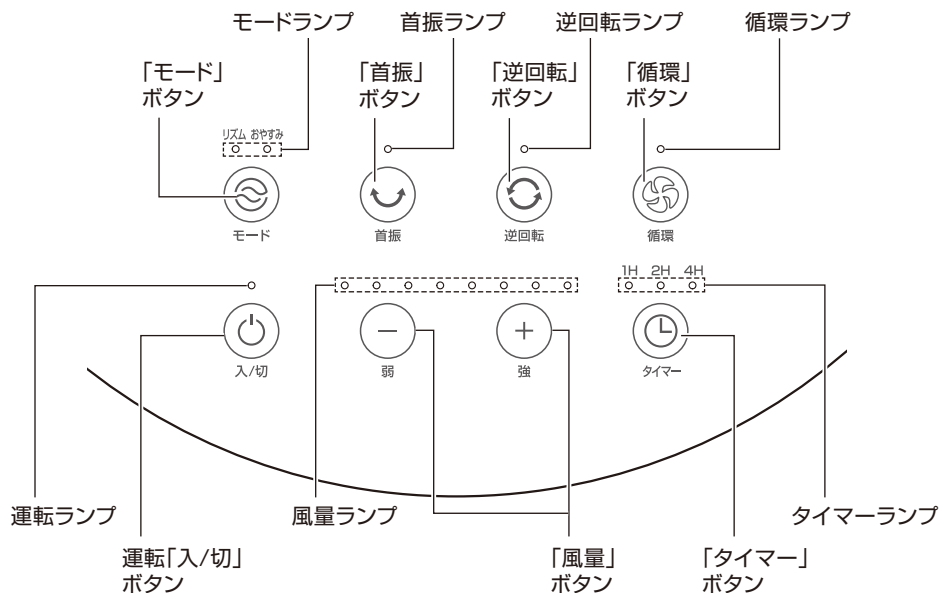
本体:操作部拡大図
